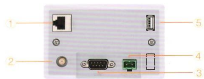
◎ 接口图
