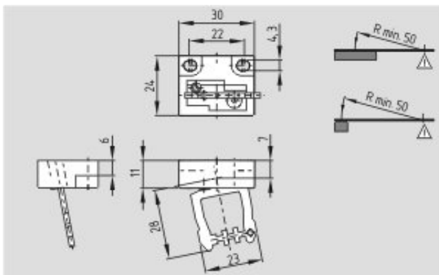
尺寸图 (操动件)
