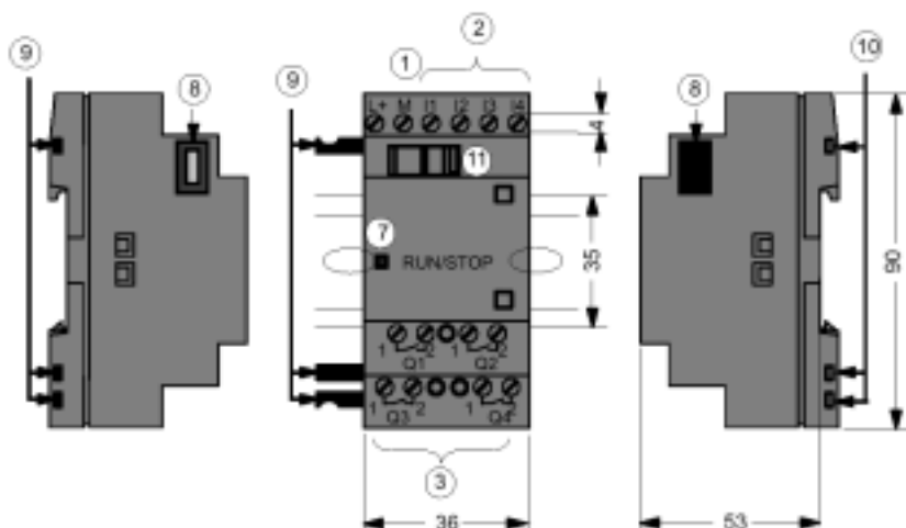
LOGO! 扩展模块 (例如: DM8 12/24 R)
