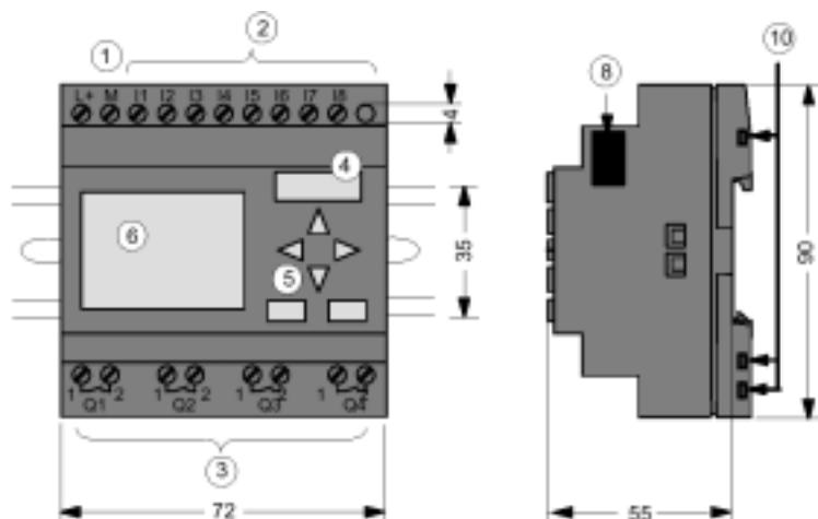
LOGO! 基本型 (例如: 12/24 RC)
