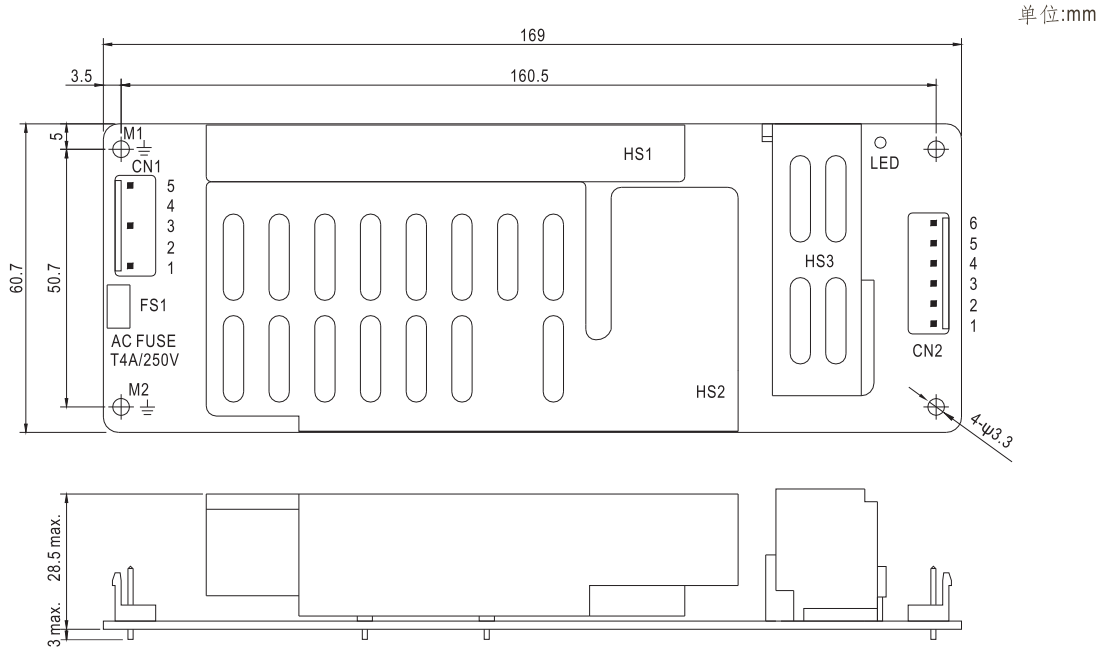
交流输入连接器(CN1): JST B5P-VH或同等级品
