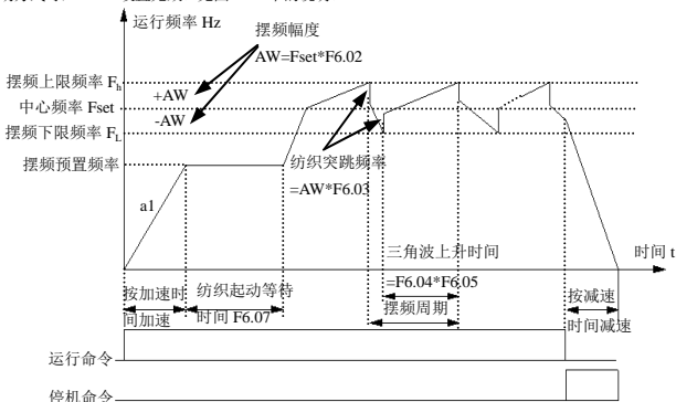
图 6-37 摆频示意图
