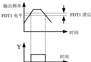
图 6-35 频率水平检测示意图
