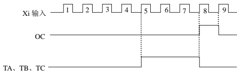
图 6-36 设定计数值给定和指定计数值给定示意图
