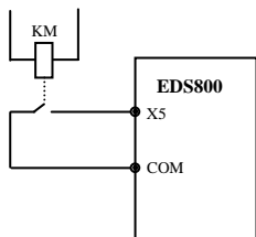
图 6-28 外部设备故障常开输入示意图
