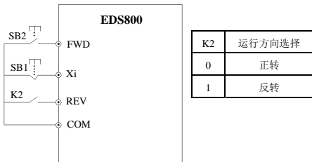
图 6-32 三线式运转模式 2
