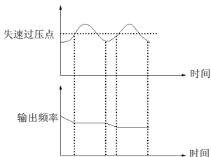
图 6-40 过压失速功能
