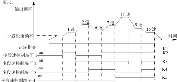
图 6-26 多段速运行示意图
