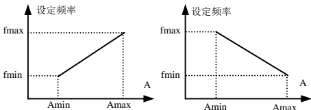
(1)正作用特性
