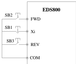
图 6-31 三线式运转模式 1
