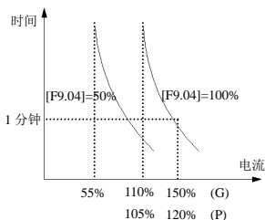
图 6-38 电子热继电器保护
