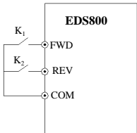
图 6-30 两线式运转模式 2
