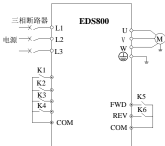
图 6-27 多段速运行接线图
