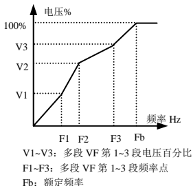
b 用户设定 V/F 曲线一般形式
