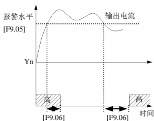
图 6-39 过载报警
