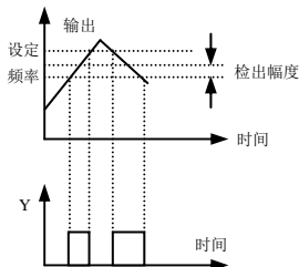
图 6-34 频率到达信号输出示意图
