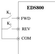
图 6-29 两线式运转模式 1
