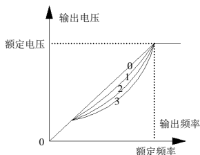
图 6-5 a V/F 曲线
