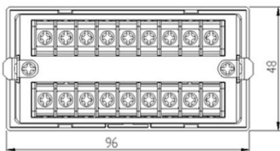
后视图
