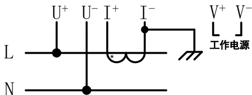
(2) 仪表端子定义
