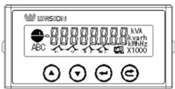
正视图
