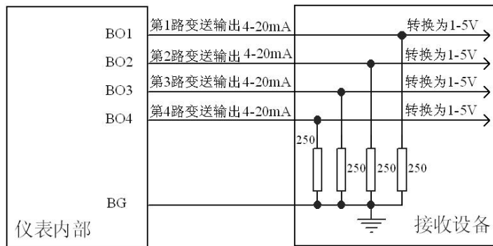
图 4.2 电流型变送输出
