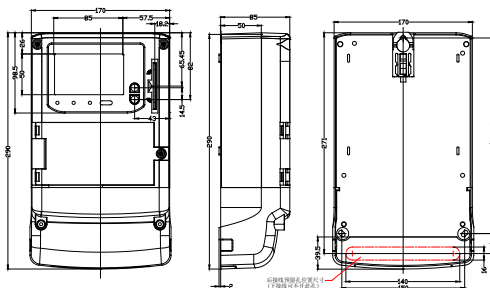
图 1: 安装尺寸图
