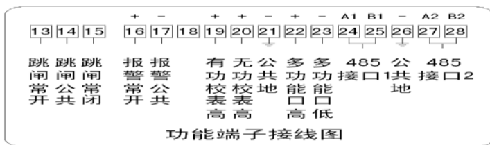
图 3：辅助端子排列图
