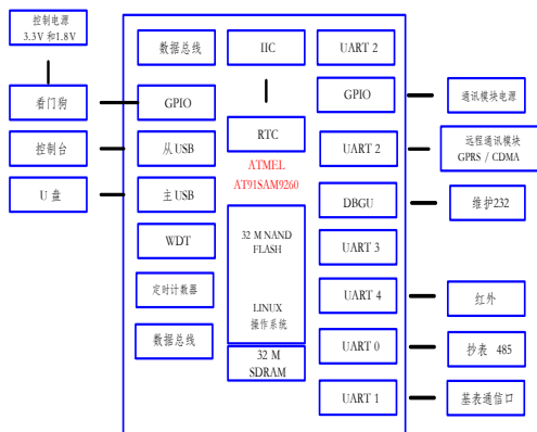
图 2-1 原理简图
