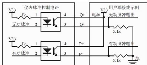
脉冲输出示意图
