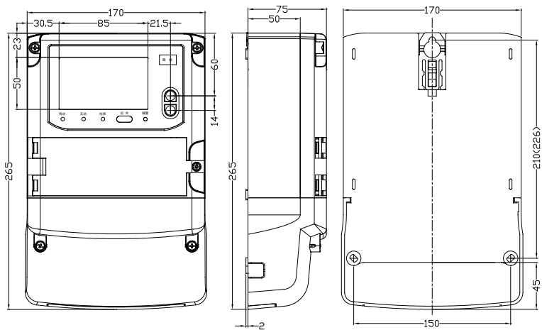
图 3：安装尺寸图
