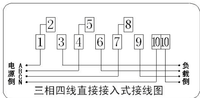
图 4：接线图
