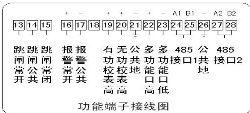
图 7：辅助端子排列图
