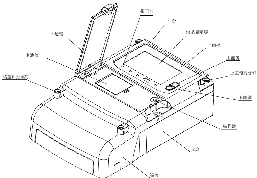
图 2：外形布局图
