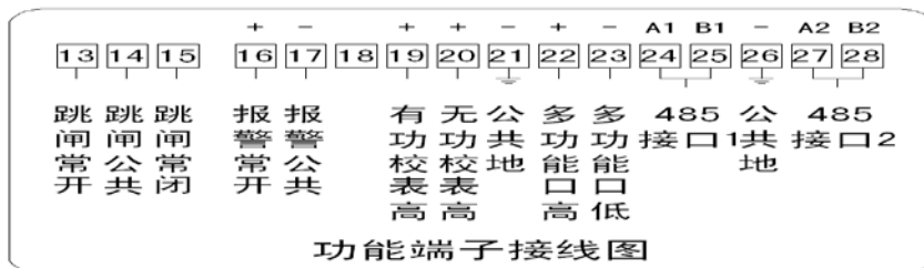
图 3: 辅助端子排列图
