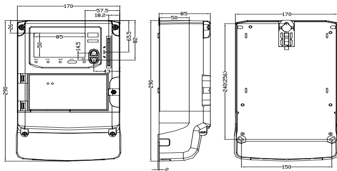
图 1: 安装尺寸图
