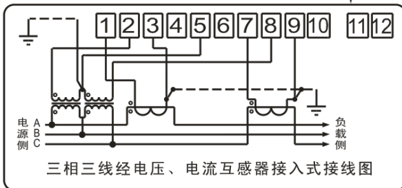
图4：接线图
