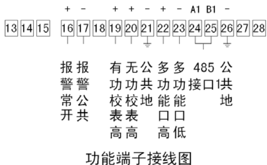
图 7C: 内继电器电能表单 485 辅助端子排列图
