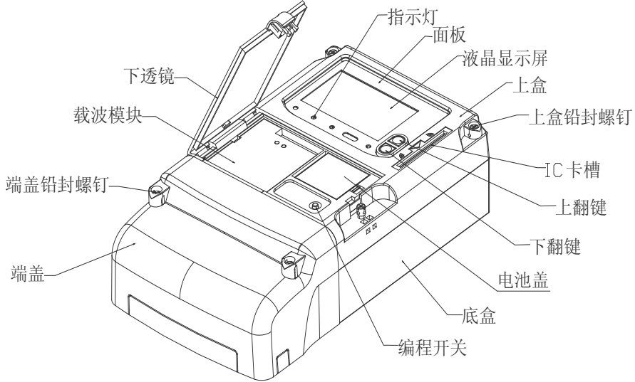
图 2：外形布局图
