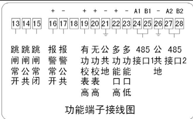
图 7：外置继电器电能表辅助端子排列图
