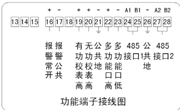
图 8：内置继电器电能表辅助端子排列图
