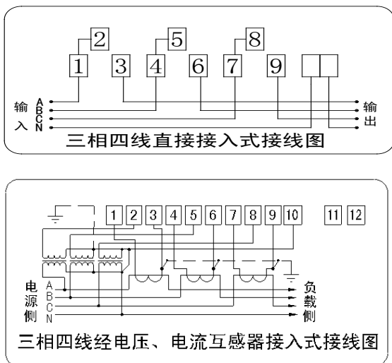
图 4：接线图
