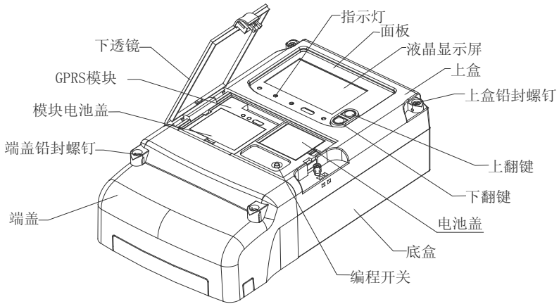
图 2：外形布局图
