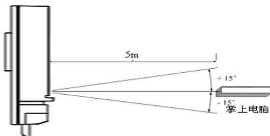
图 10 现场红外设置示意图
