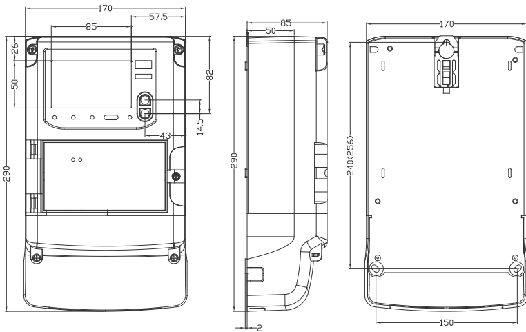
图 3：安装尺寸图
