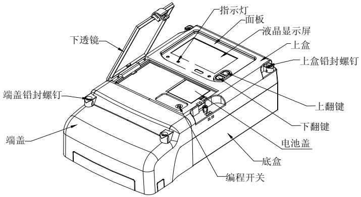
图 2：外形布局图
