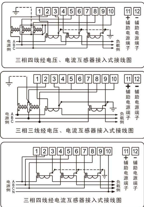
图 4：接线图
