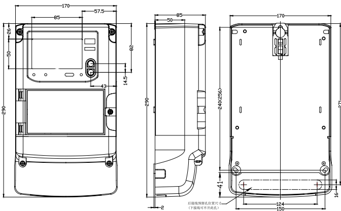
图 3：安装尺寸图
