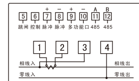
图2: 经互感器接入式
