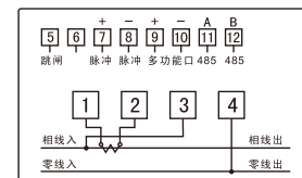
图4: 经互感器接入式(5脚输出220V信号)
