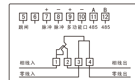
图3: 直接接入式(5脚输出220V信号)
