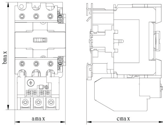
△ GSC1-40/50/65/80/95+JRS4-40/80d
