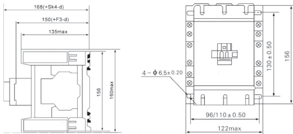
△ GSC1-115/150
