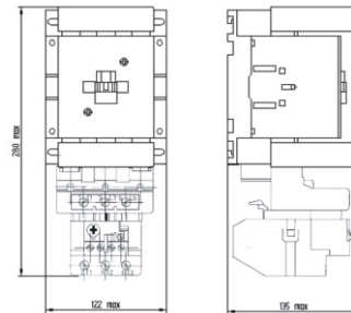
△ GSC1-115/150+JRS4-140d
