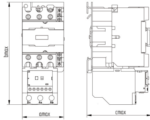
△ GSC1-40/50/65/80/95+GSR3-40/95
