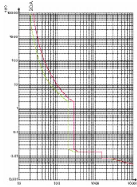
20A脱扣曲线
