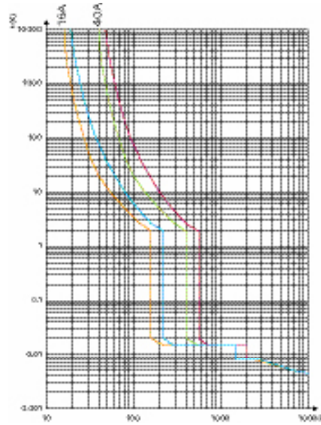
16A, 40A脱扣曲线
