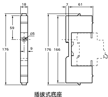
插拔式底座
