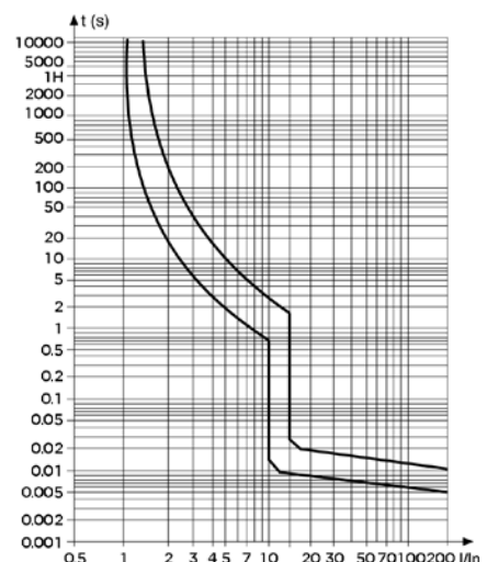
C65L D型曲线
