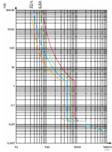
32A, 63A脱扣曲线
