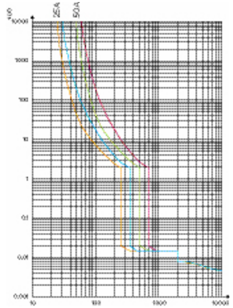
25A, 50A脱扣曲线
