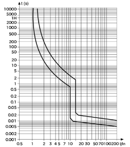
C65N/H D型脱扣曲线
